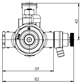
Afmetingen 28 0352 / 28 0353
