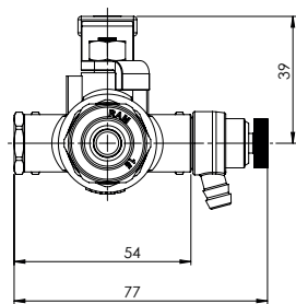
Afmetingen 28 0350 / 28 0351
